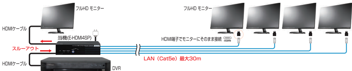
接続図
