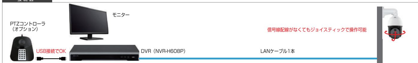
接続図
