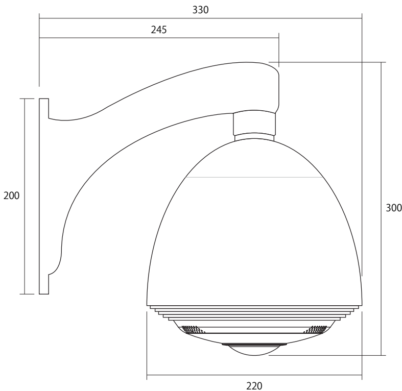
製品図
